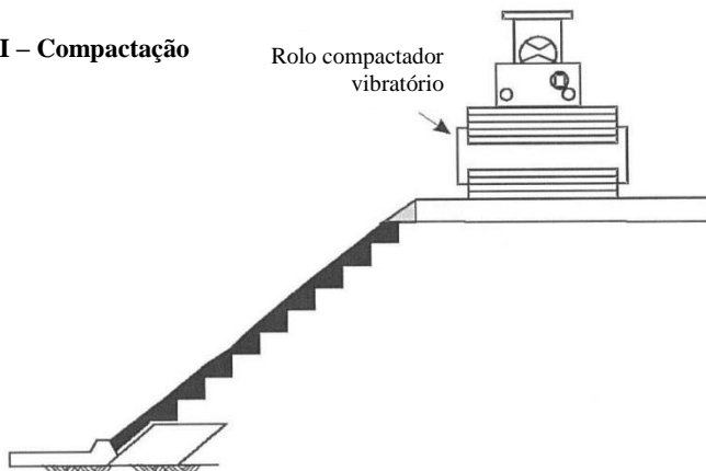
Figura 18. Construção da borda do talude de montante com material 2 A.
