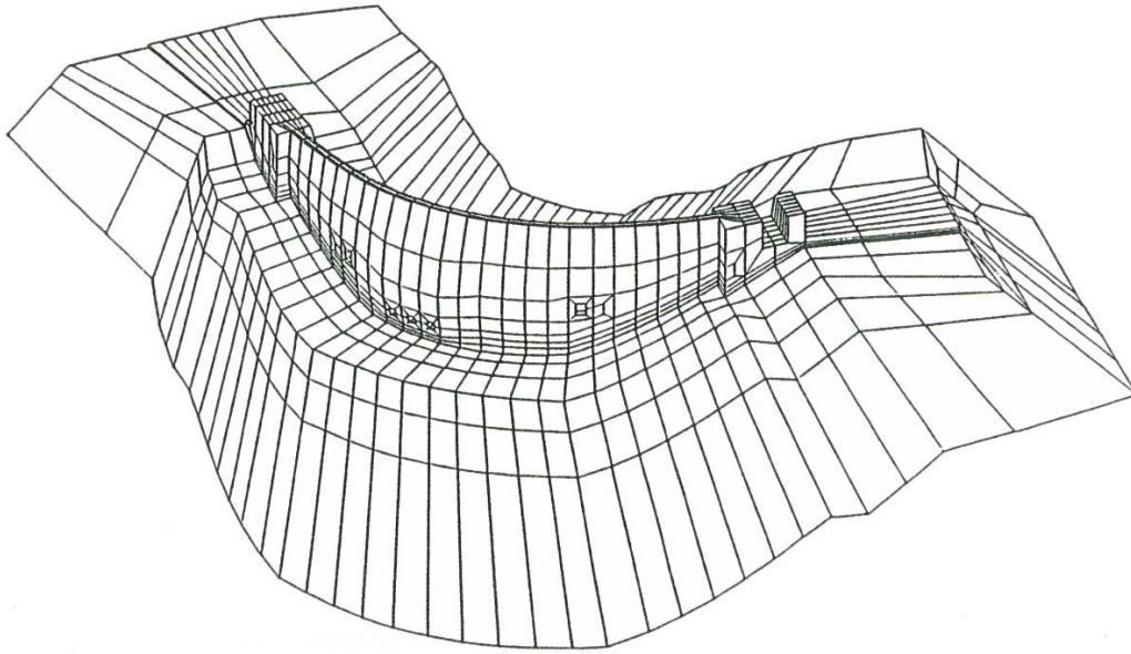
Modelo de elementos finitos– vista de montante
