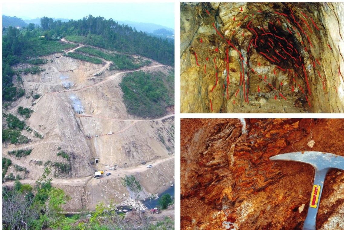
Figura 1. Modelo geológico 2D de uma barragem de concreto gravidade (Barragem de Ribeiradio, Portugal). (Fonte: OLIVEIRA et al., 2006)
