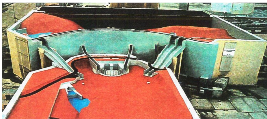
Figura 30. Modelo hidráulico utilizado no estudo do vertedouro de superfície e dos descarregadores de meio fundo de uma barragem em arco. (Fonte: LNEC, EDIA)
