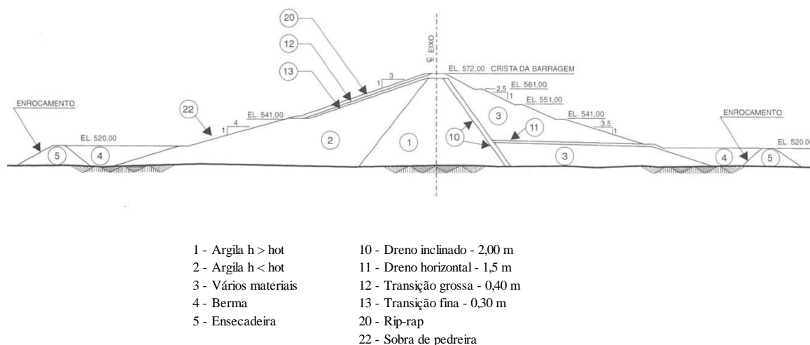
Figura 11. Seção típica de uma barragem de terra zonada. Barragem de Três Marias, MG – seção no leito do rio. (Fonte: CRUZ, 2004)
