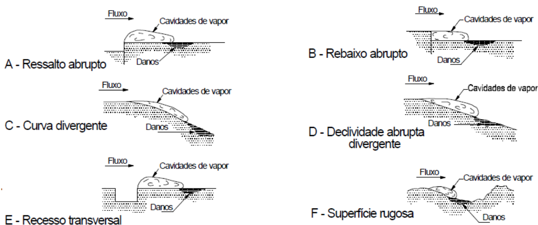
Figura 40. Tipos de irregularidades de superfícies de concreto e zonas de erosão por cavitação. (Fonte: INAG, 2001)
