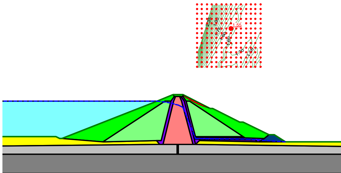
Figura 15. Análise de estabilidade pelo método de Bishop Modificado. Situação de percolação estável.
