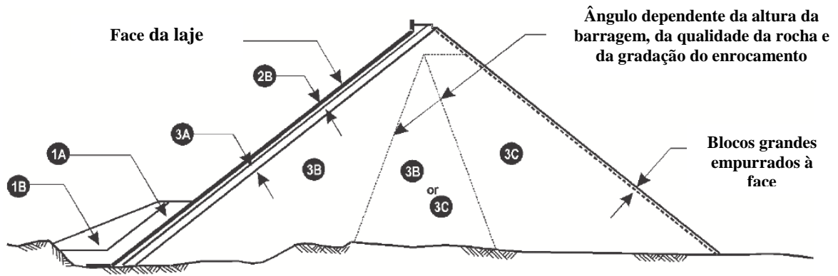
Seção da barragem
