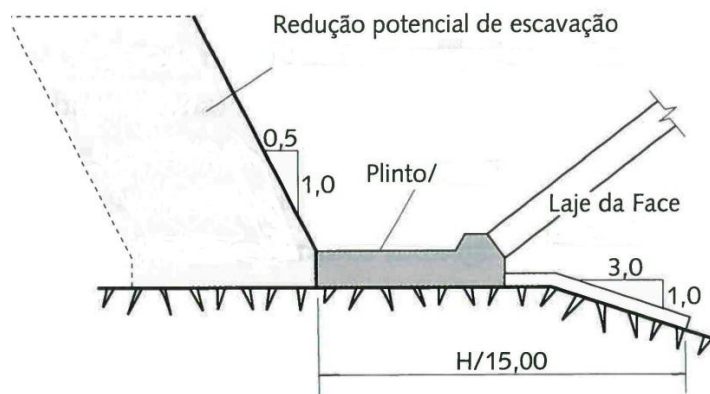
Figura 19. Seção da laje do plinto de montante e jusante (interno).
