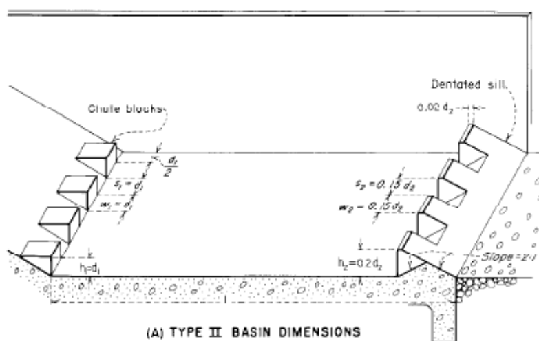
Figura 32. Bacia de dissipação do Tipo II. (Fonte: USBR, 1973)
