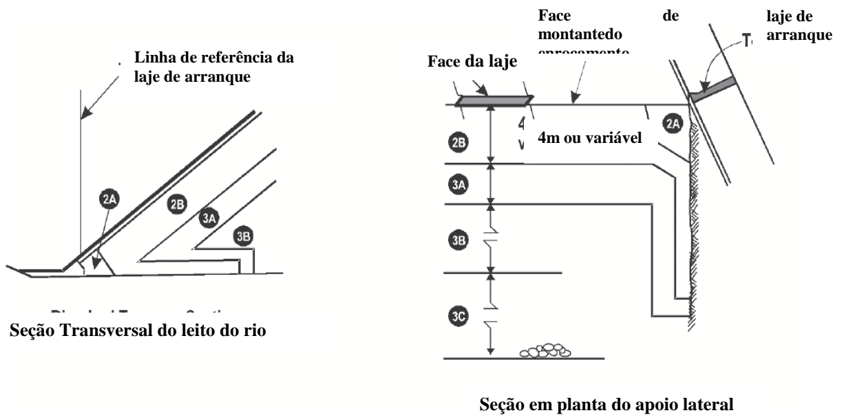
Seção da barragem
