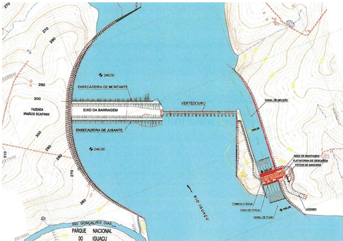
Figura 9. Desvio do rio em diversas fases. 2ª Fase. Desvio pelo vertedor, com uso de ensecadeira incorporada de montante e de jusante. UHE Baixo Iguaçu, PR. (Fonte: ROCHA, 2006)
