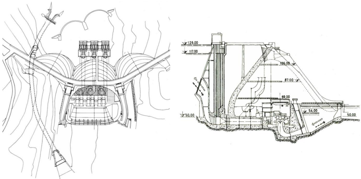
Figura 25. Barragem da Aguieira, Portugal (arcos múltiplo de grande vãos de dupla curvatura, com 89 m de altura máxima, concluída em 1981). (Fonte: CNPGB, 1992)
