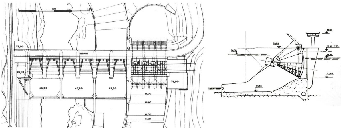
Figura 26. Barragem de Fratel, Portugal (barragem de soleira vertente, com 43 m de altura máxima, concluída em 1973). (Fonte: CNPGB, 1992)
