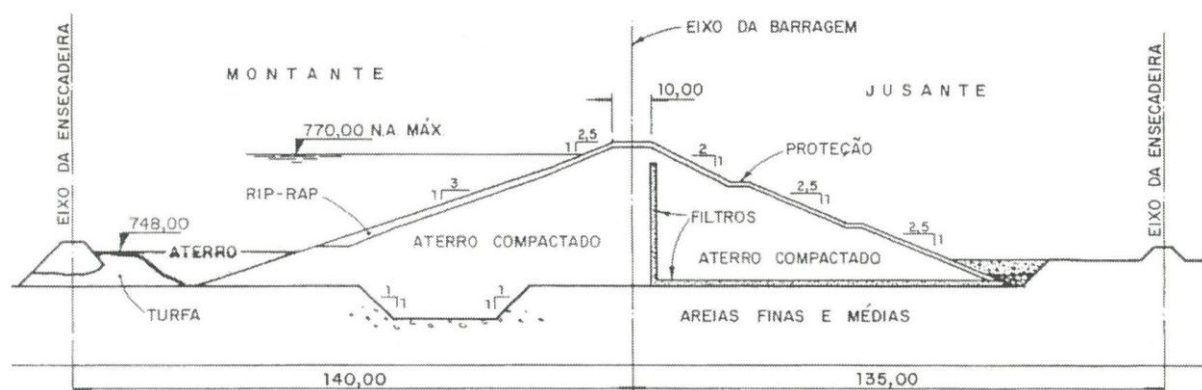
Figura 10. Seção típica de uma barragem de terra homogênea. Barragem de Ponte Nova, SP. (Fonte: CRUZ, 2004)
