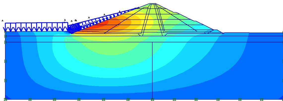
Figura 16. Análise de tensões deformações. Modelação do primeiro enchimento do reservatório. Deslocamentos horizontais.
