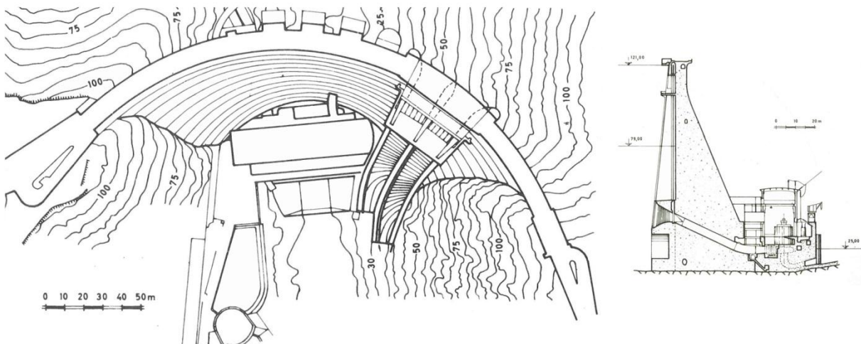
Figura 24. Barragem do Castelo do Bode, Portugal (arco-gravidade com 115 m de altura máxima, concluída em 1951). (Fonte: CNPGB, 1992)
