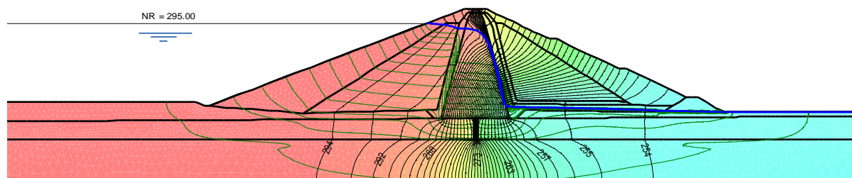
Figura 14. Análise de percolação em regime permanente pelo método dos elementos finitos (linhas equipotenciais).
