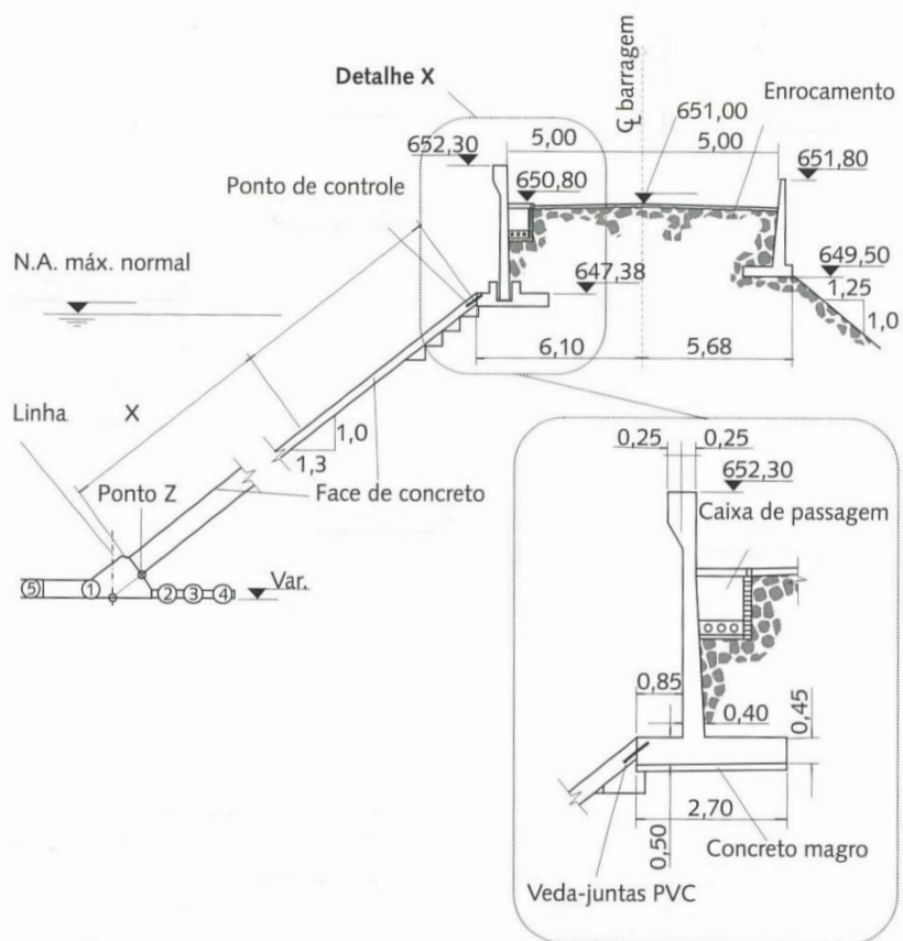
Figura 23. Detalhe do muro da crista e da junta de expansão no contato laje-fundação do muro da barragem de Barra Grande, RS/SC. (Fonte: CRUZ; MATERÓN; FREITAS, 2009)
