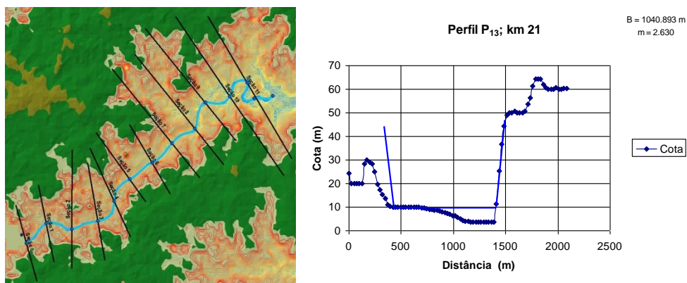
Figura 43. Caracterização topográfica do vale a jusante. a) seções transversais do vale e a altimetria do SRTM, b) ajustamento de seções regulares às seções naturais.
