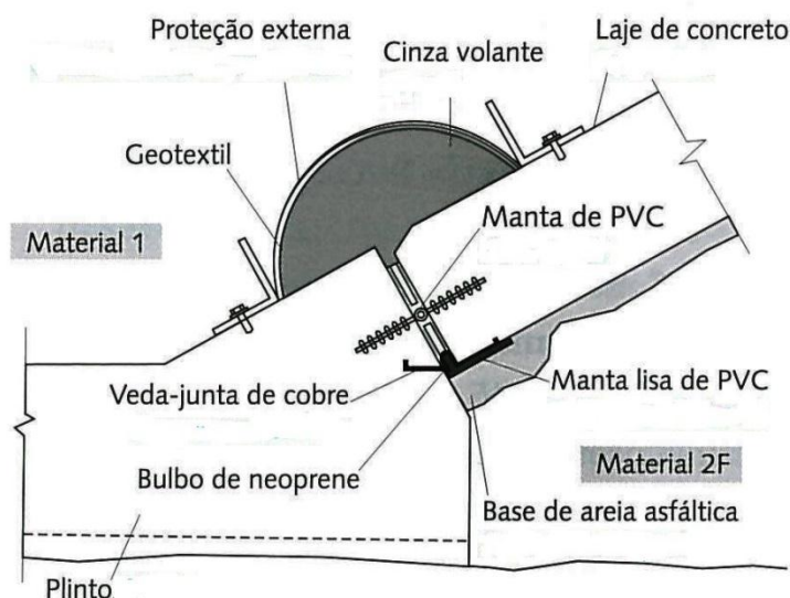
Figura 21. Junta perimetral. Utilização de cinza volante em alternativa ao mastique. Barragem de Aguamilpa, México. (Fonte: CRUZ; MATERÓN; FREITAS, 2009)
