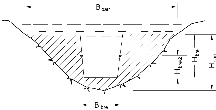
Figura 42. Esquema da seção típica da brecha em barragens de aterro.
